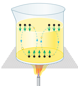
Figura 9. Correntes de convecção num líquido em aquecimento.
