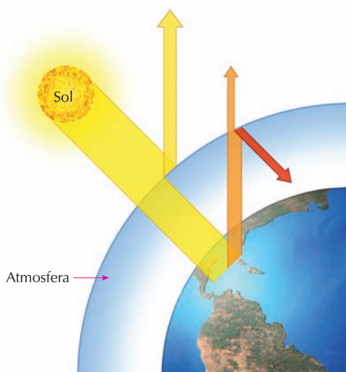
Figura 13. Esquema do efeito estufa
