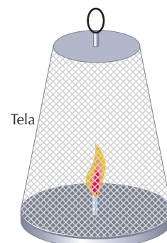
Figura 8. Lâmpada de Davy.
