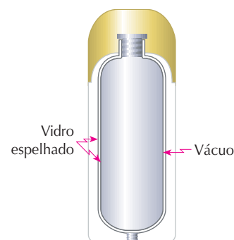
▲ Figura 14. Garrafa térmica.
