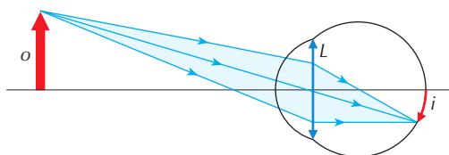
« Figura 16. Formação da imagem no olho humano.
