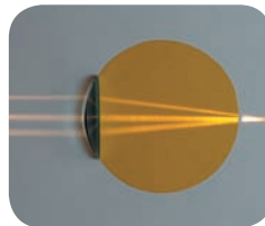
Figura 22. O hipermetrope deve realizar esforço de acomodação para ver nitidamente objetos no infinito.
