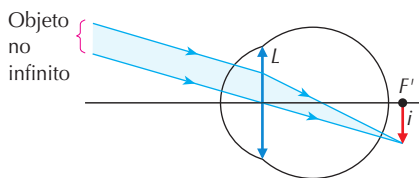
Figura 22. O hipermetrope deve realizar esforço de acomodação para ver nitidamente objetos no infinito.
