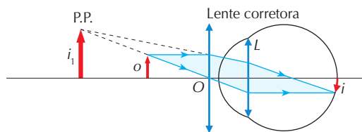
Figura 24. (A) A lente corretora forma do objeto a 25 cm uma imagem i_1 no ponto próximo (P.P.) do olho hipermetrope. (B) Simulação da influência da lente corretora sobre o olho hipermetrope.
