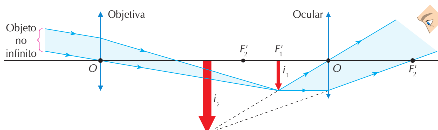
Figura 9. Formação da imagem na luneta astronômica.
