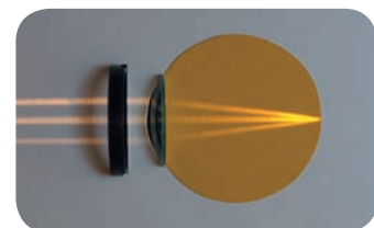
Figura 24. (A) A lente corretora forma do objeto a 25 cm uma imagem i_1 no ponto próximo (P.P.) do olho hipermetrope. (B) Simulação da influência da lente corretora sobre o olho hipermetrope.
