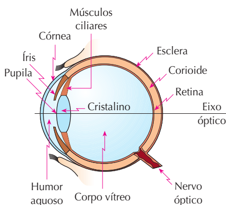
« Figura 14. Corte esquemático do olho humano.
