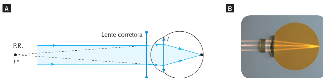
▲ Figura 21. (A) A lente corretora forma do objeto no infinito uma imagem no ponto remoto (P.R.) do olho míope. (B) Montagem simulando a influência da lente corretora sobre o olho míope.
