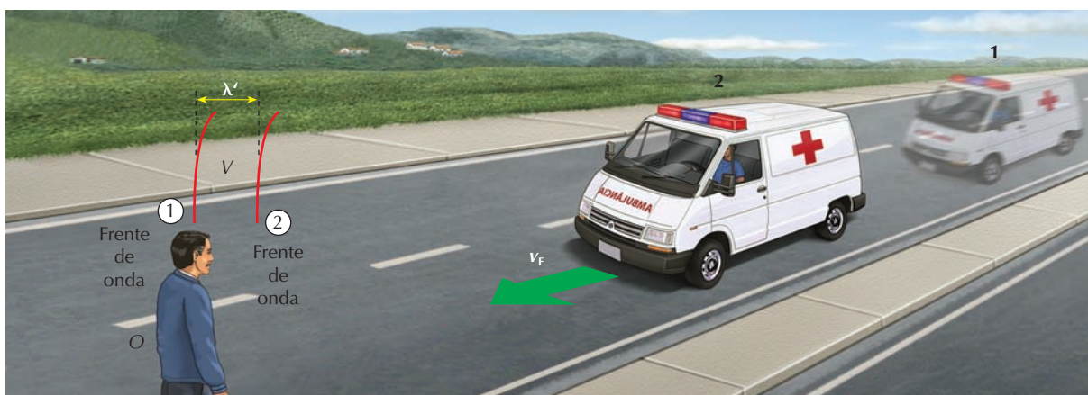
▲ Figura 13. O observador parado recebe o som emitido pela ambulância com frequência aparente f' maior que a frequência f real.
