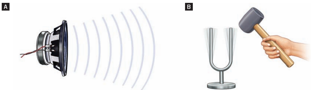
▲ Figura 2. Ondas sonoras podem ser produzidas por objetos vibrando, como o diafragma de um alto-falante (A) ou um diapasão (B).
