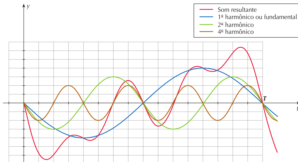
Figura 5. Composição dos sons emitidos por um instrumento.
