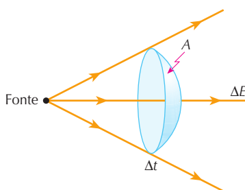
Figura 4. A intensidade física de uma onda é a medida da energia que atravessa uma superfície pela área da superfície na unidade de tempo.
