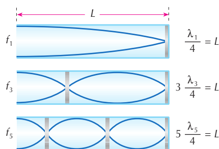
Figura 10. Modos naturais de vibração de uma coluna de ar em um tubo fechado numa extremidade. As regiões mais escuras, onde a pressão do ar é maior, correspondem aos nós.
