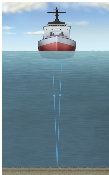
Esquema do sonar.
