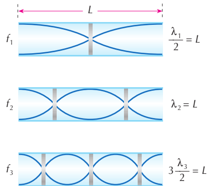
« Figura 12. Modos naturais de vibração de uma coluna de ar num tubo aberto. A natureza longitudinal é sugerida pelas regiões mais escuras. Onde a pressão do ar é maior formam-se os nós.
