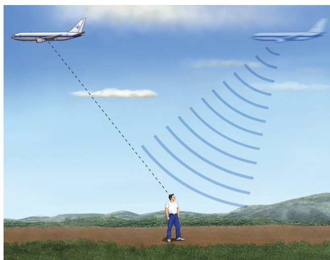
◀ Figura 3. O som se propaga no ar com velocidade pequena quando comparada com a velocidade da luz.
