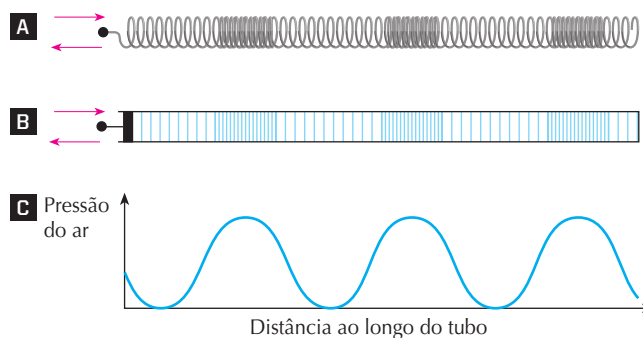
Figura 1. Onda longitudinal estabelecida em uma mola (A) e no ar dentro de um tubo (B). O gráfico (C) indica a pressão do ar ao longo do tubo.
