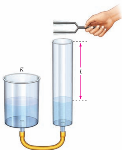
Figura 9. Ressonância de uma coluna de ar com um diapasão.
