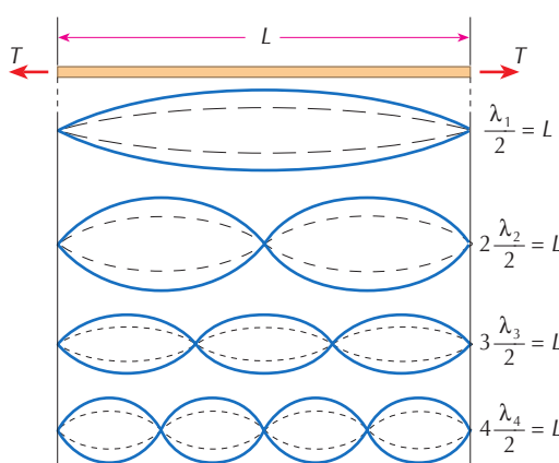
« Figura 8. Ondas estacionárias em uma corda vibrante.
