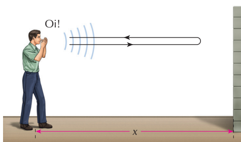
Figura 6. Para haver eco, deve-se ter x > 17 m.
